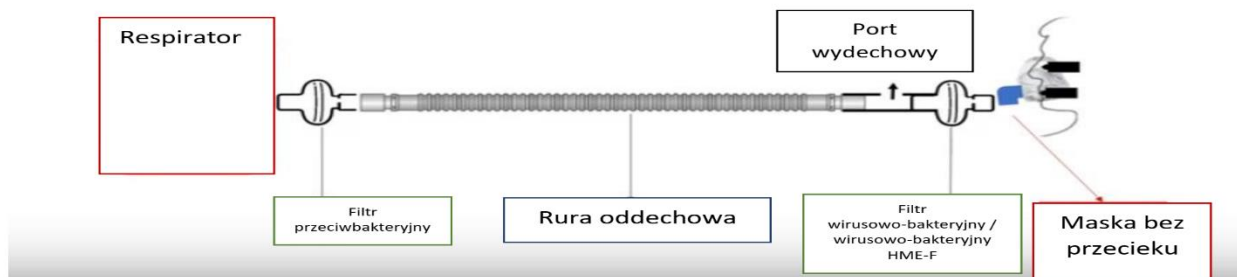
Rys.3. Przykłady konfiguracji NIV z maską, filtrem, portem wydechowym – układ z pojedynczą rurą oddechową
